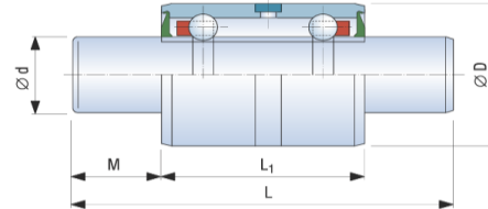
Typ / Type: 76-3-7, 76-3-7KK
